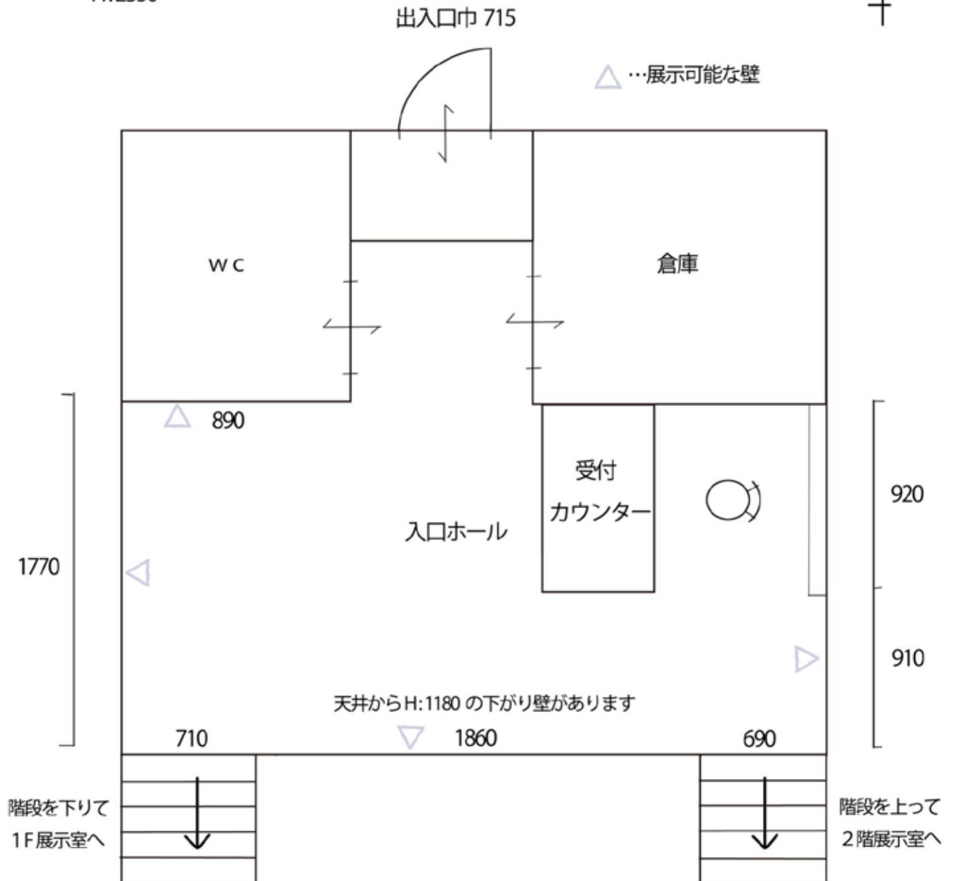
入口ホール平面図 H:2330
